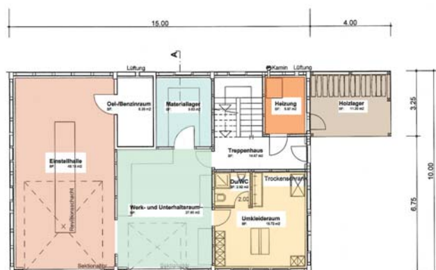
Grundriss Erdgeschoss
