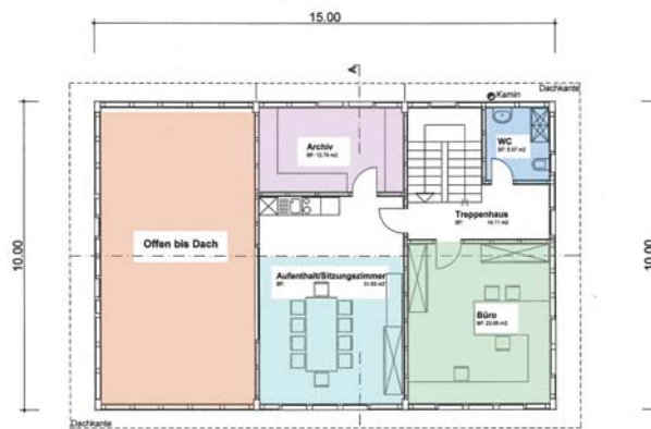
Grundriss Obergeschoss
